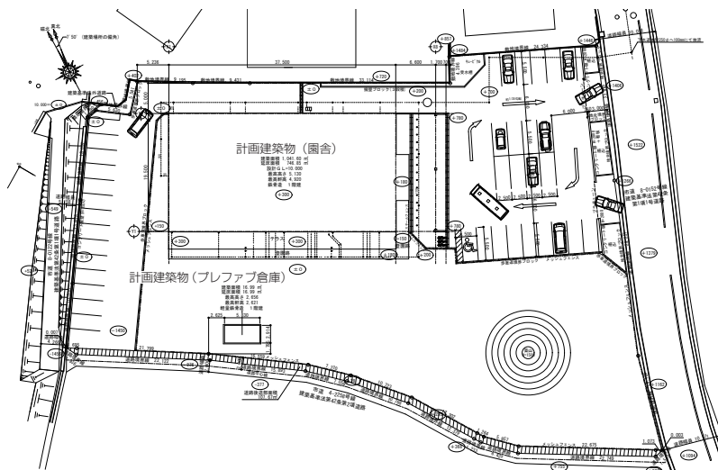
配置図
