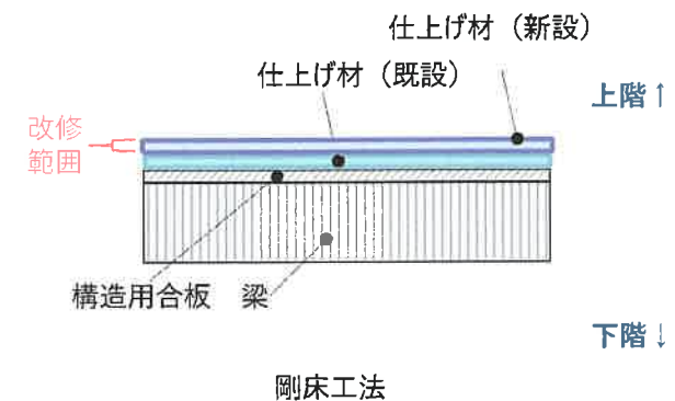
図2 横から見た断面図
