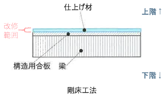
図1 横から見た断面図
