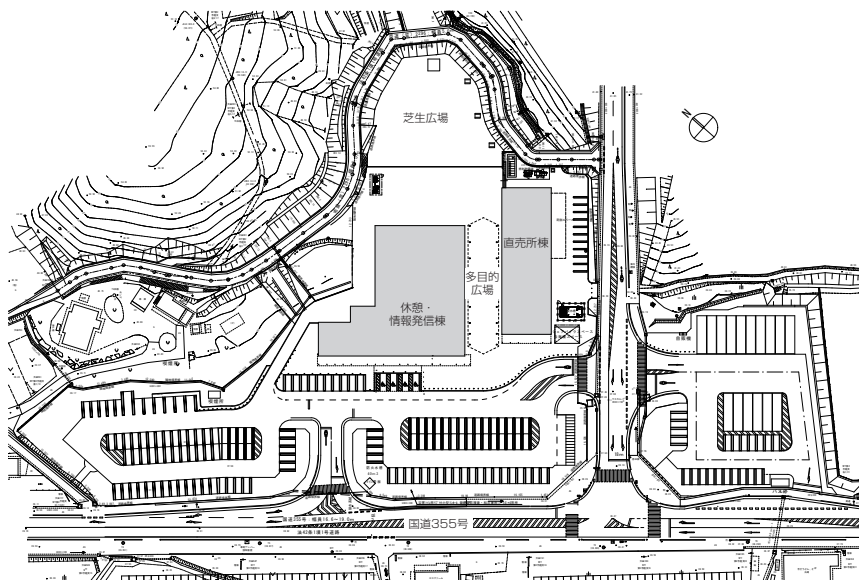
配置図
